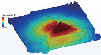
TF-QFLUX软件采用LEVEL湍流模型和Boussinesq假设模拟某驾驶辅助系统ADAS散热特性和周围空气的自然对流：部件表面温度云图分布
