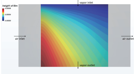
散热器相变仿真: 高温蒸汽遇冷空气发生冷凝及在管壁上形成液膜, 图为液膜厚度分布 (相变和液膜模型)
