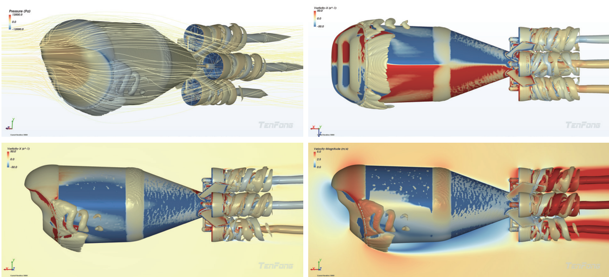
深海潜航器水动力特性仿真
