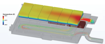
TF-QFLUX软件采用SST k-w湍流模型、流固耦合传热模拟IGBT水冷散热：管内流线形态与固体表面温度云图分布
