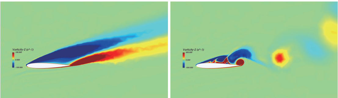
NACA0012翼型绕流: AOA=15°, 展向涡量云图 (湍流模型: URANS)
