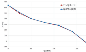
TF-QFLUX软件采用IDDES湍流模型、FW-H方法和非定常计算模式，模拟电子系统风扇功率特性和远场噪声：Q等值面和等值面上速度云图分布（左）、风扇P-Q曲线计算值与某对标软件对比（中）、某测点风噪频谱特性计算值与某对标软件对比（右）
