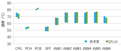
TF-QFLUX软件采用LEVEL湍流模型、热辐射模型和流固紧耦合计算模式，模拟机箱散热特性：机箱内流场结构（流线分布）和散热件表面温度分布（左）、部件表面温度分布范围计算值与参考值对比情况（右）
