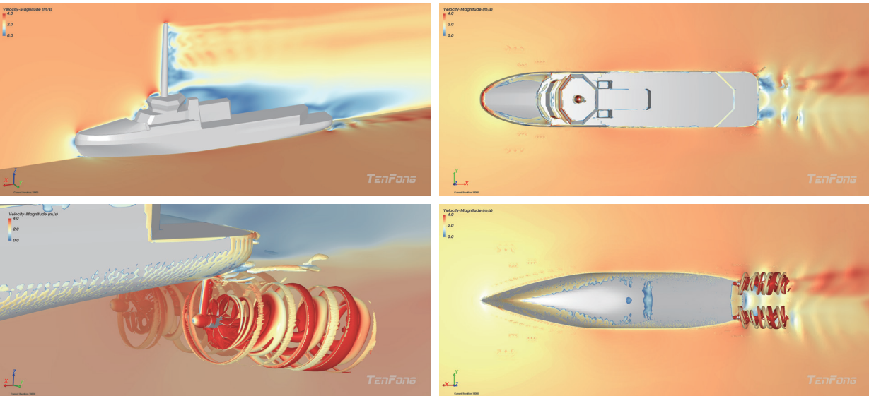
船舶水动力特性仿真
