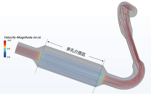
汽车排气管催化器流动仿真: 管内流线分布 (多孔介质模型)
