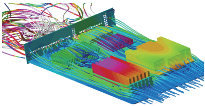
TF-QFLUX软件采用LEVEL湍流模型、热辐射模型和流固紧耦合计算模式，模拟机箱散热特性：机箱内流场结构（流线分布）和散热件表面温度分布（左）、部件表面温度分布范围计算值与参考值对比情况（右）
