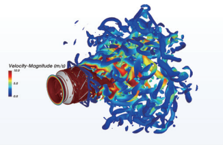
TF-QFLUX软件采用IDDES湍流模型、FW-H方法和非定常计算模式，模拟电子系统风扇功率特性和远场噪声：Q等值面和等值面上速度云图分布（左）、风扇P-Q曲线计算值与某对标软件对比（中）、某测点风噪频谱特性计算值与某对标软件对比（右）
