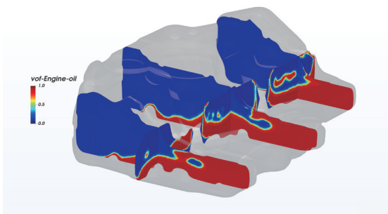
油箱晃动: 不同截面油相体积分分布 (VOF模型)
