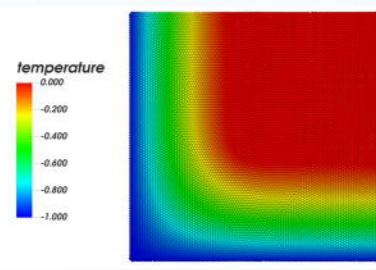
金属相变
