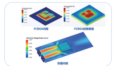
芯片电子热设计
