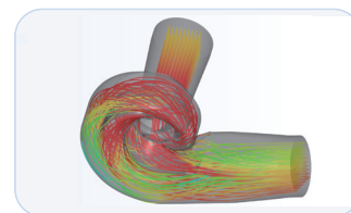
高速离心泵流致振动噪声分析
