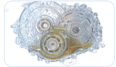
齿轮润滑冷却仿真
