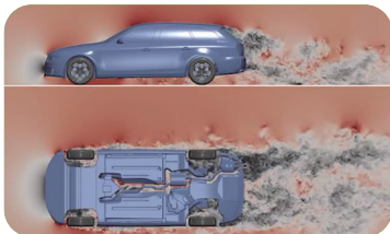
高精度瞬态汽车空气动力学仿真
