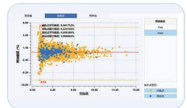
光学器件代理模型精度评估
