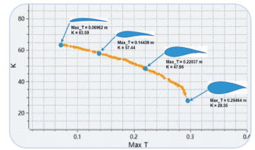
航空翼型多目标优化
