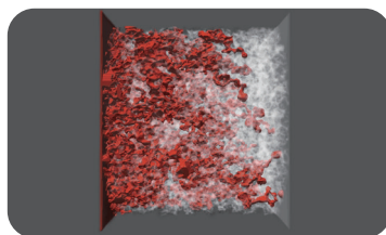
油气开采-岩心渗油动态仿真
