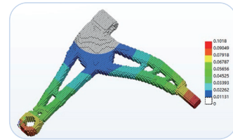
增减材一体化优化设计
