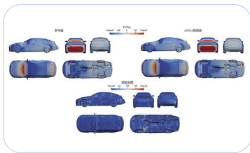
“秒级”汽车空气动力学快速设计迭代
