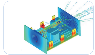
机箱热仿真
