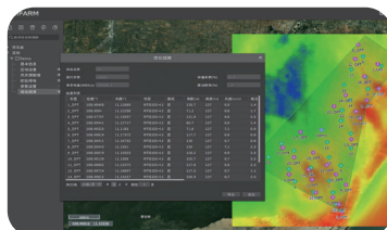
风场排布优化
