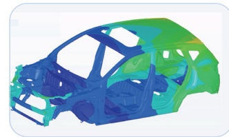
车身扭转刚度分析
