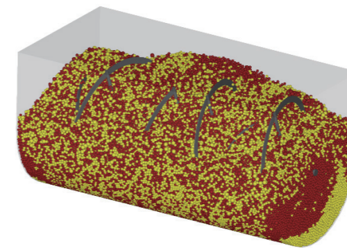
Ribbon混合机
