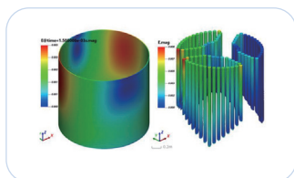
电锅炉电场仿真
