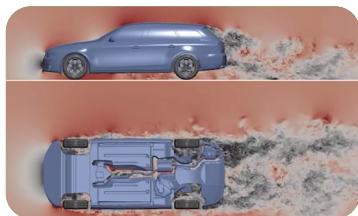
高精度瞬态汽车空气动力学仿真
