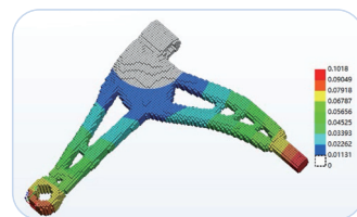
增减材一体化优化设计
