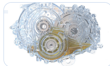
齿轮润滑冷却仿真
