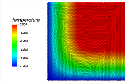
金属相变
