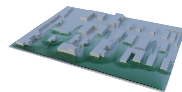
城市洪涝
