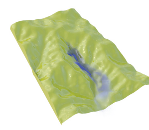
山谷洪水
