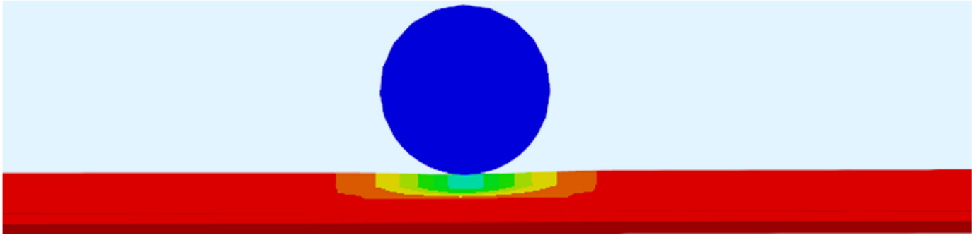
Neo-Hookean超弹模型，小球跌落
