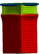
网格畸变状态下的稳定求解
