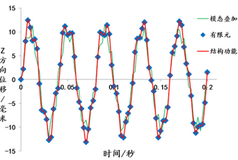
结构功能与模态叠加法结果的比较
