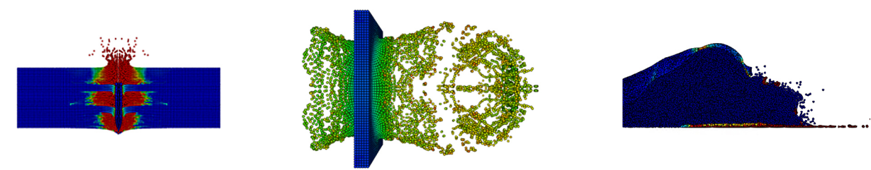
多层混凝土靶板侵彻
