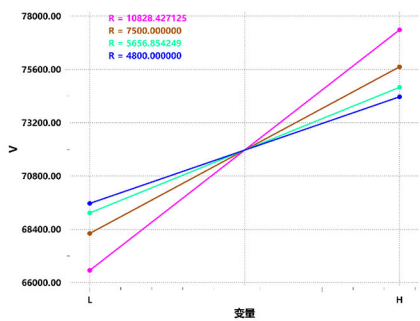
主效应分析
