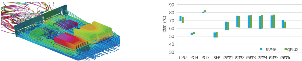
TF-QFLUX软件采用LEVEL湍流模型、热辐射模型和流固紧耦合计算模式，模拟机箱散热特性：机箱内流场结构（流线分布）和散热件表面温度分布（左）、部件表面温度分布范围计算值与参考值对比情况（右）
