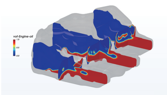
油箱晃动: 不同截面油相体积分数分布 (VOF模型)
