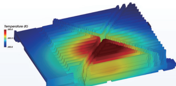
TF-QFLUX软件采用LEVEL湍流模型和Boussinesq假设模拟某驾驶辅助系统ADAS散热特性和周围空气的自然对流：部件表面温度云图分布
