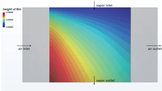
散热器相变仿真: 高温蒸汽遇冷空气发生冷凝及在管壁上形成液膜, 图为液膜厚度分布 (相变和液膜模型)
